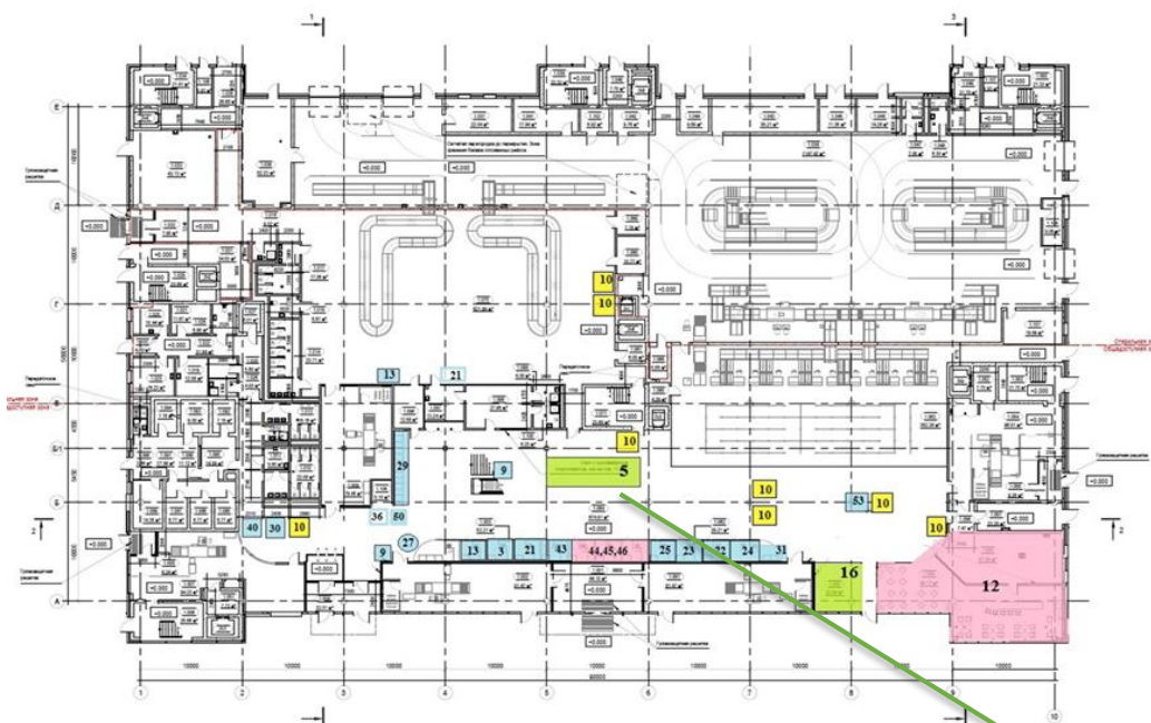
План 1-го этажа (на отм. 0.000). М 1:200
